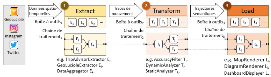
Figure 1. Chaîne de traitement des données inspirée des procédures ETL
