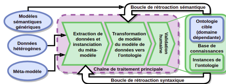
Figure 2. Cadre méthodologique pour la population d'ontologies.
