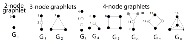
Figure 1. Représentation des 9 graphlets de 2 jusqu'à 4 nœuds
