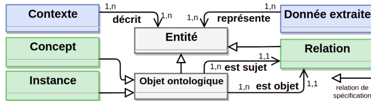
Figure 1. Métamodèle générique pour l'extraction de données hétérogènes.
